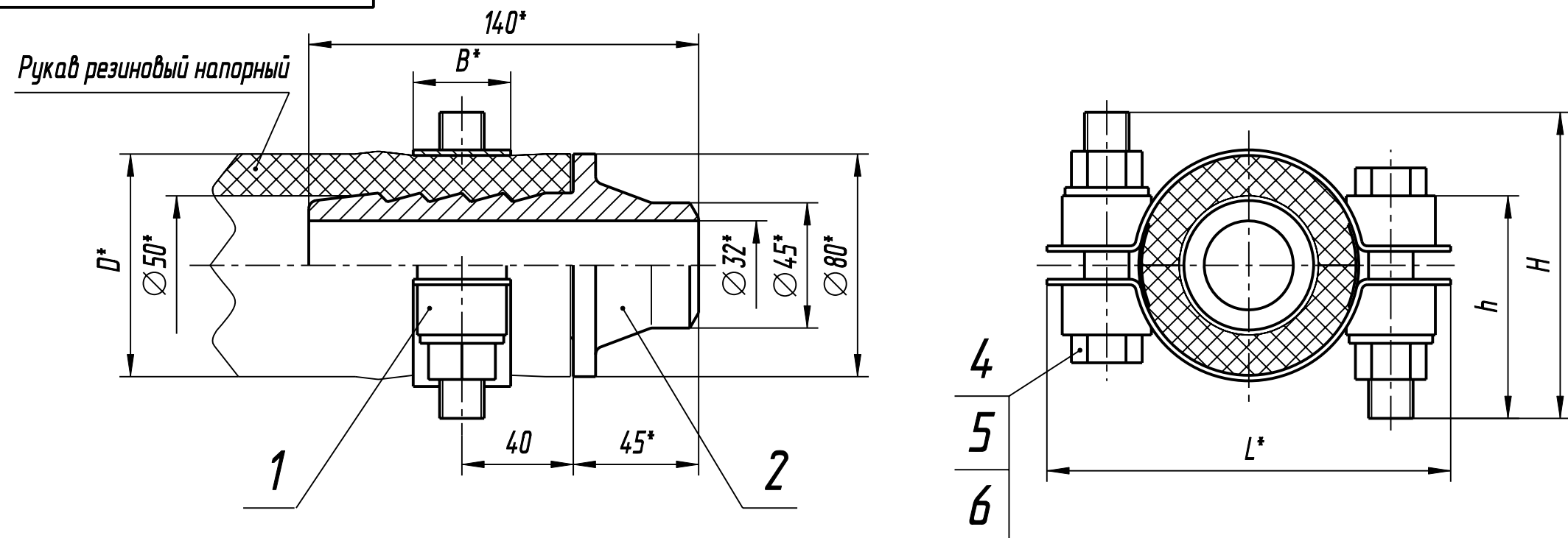
Размеры в мм
